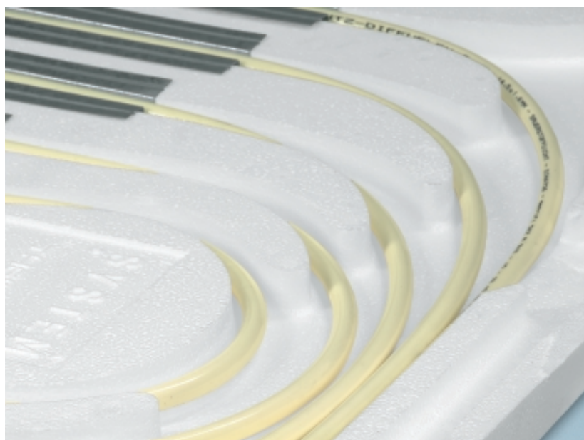
THERMOLUTZ Diffuflex-S-Heizrohr aus Polybuten
