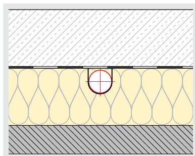
Bauart B nach DIN 18560, Teil 2
