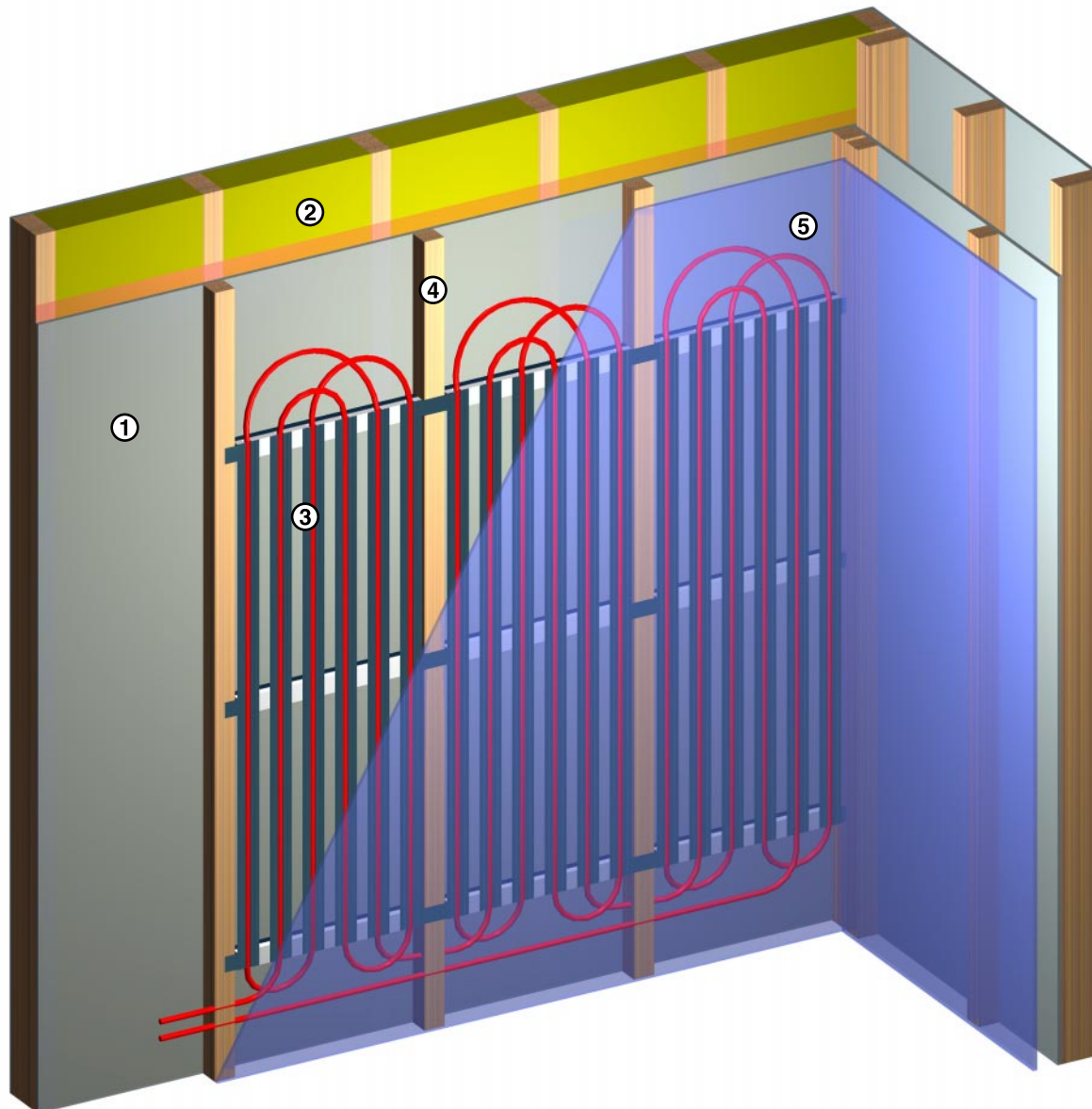
Wandheiz-Modul ACULAR-M in Installationsebene Holzständerwand
